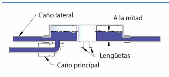
Vista de corte del contenedor de distribución de agua
