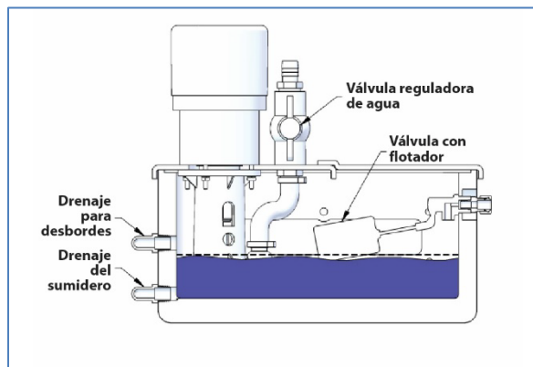
Vista de corte del sumidero de agua
